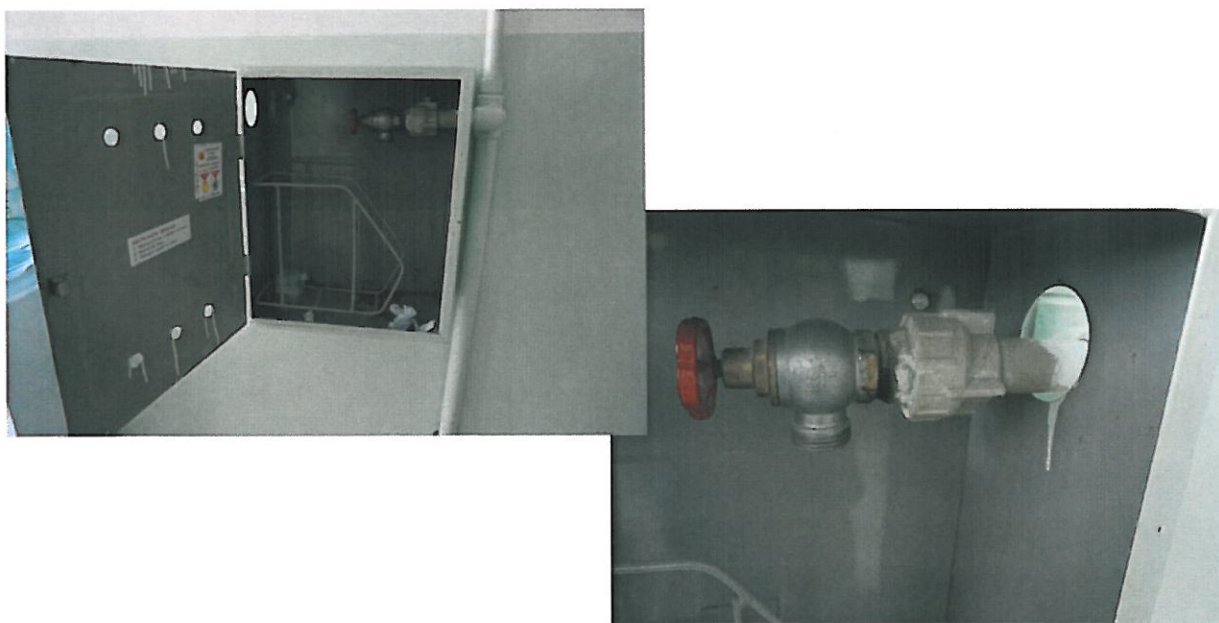
fot. 9. Wewnętrzna instalacja hydrantowa - przykładowe fotografie (opracowanie własne)
